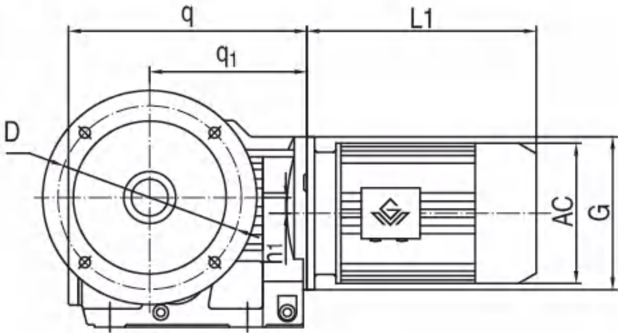
GKHF39-159 安装结构尺寸
