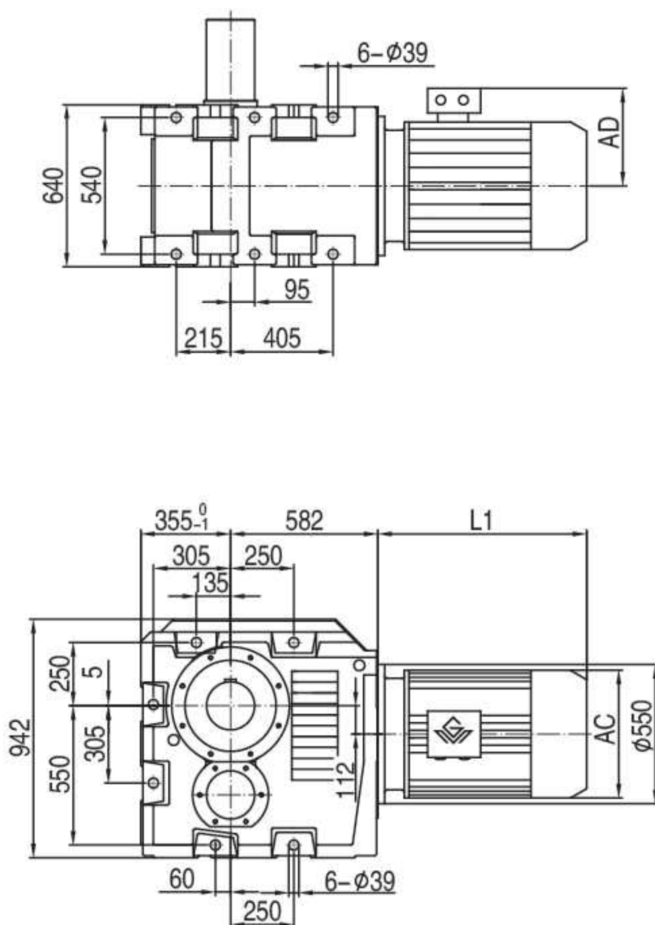
GK189 安装结构尺寸
