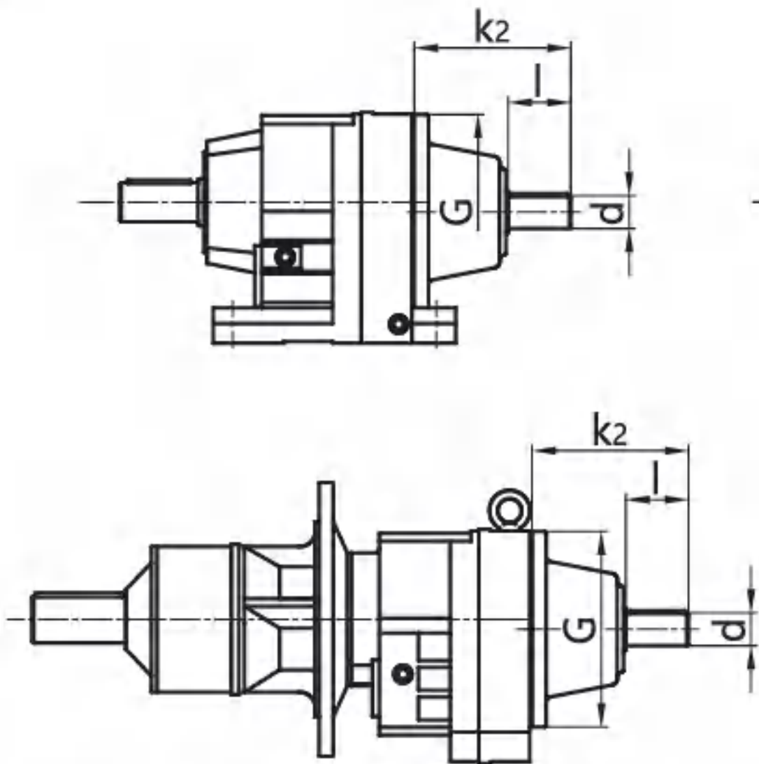
GR..29-179AD1-8 安装结构尺寸
