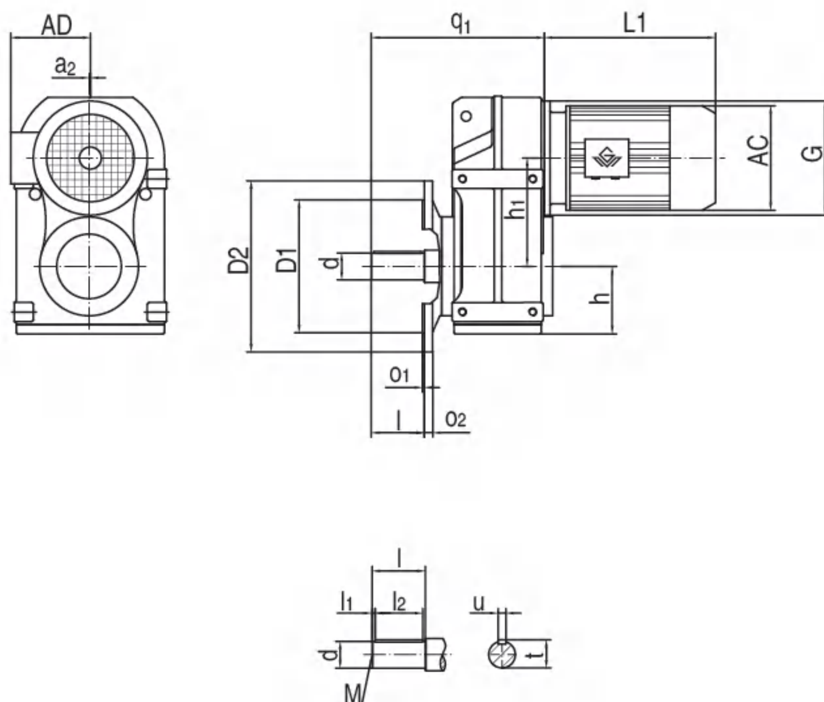
GFF39-159 安装结构尺寸
